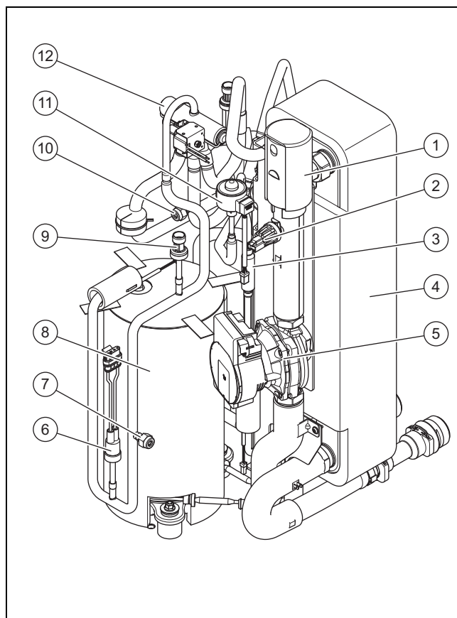
1 Быстродействующий воздухоотводчик 2 Датчик давления в отопительном контуре 3 Фильтр 4 Конденсатор 5 Насос системы отопления 6 Реле давления на участке высокого давления 7 Сервисный штуцер на участке высокого давления 8 Компрессор 9 Датчик давления на участке высокого давления
