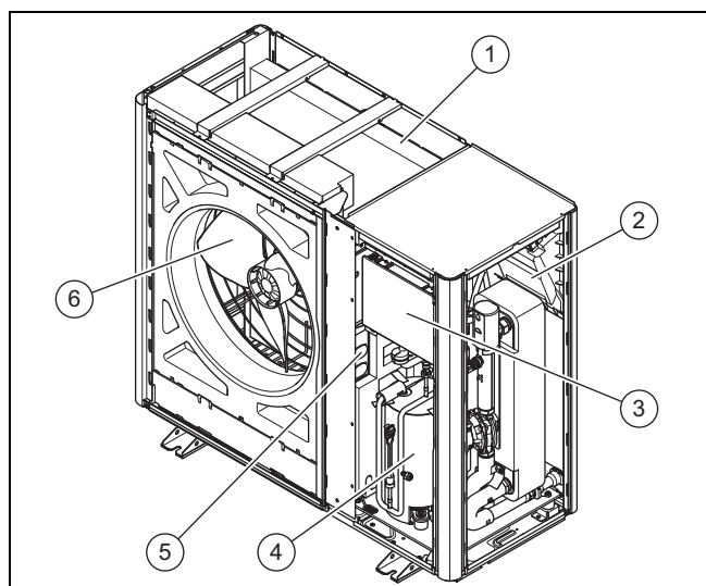
1 Испаритель 2 Электронная плата INSTALLER BOARD 3 Электронная плата HMU 4 Компрессор 5 Узел INVERTER 6 Вентилятор
