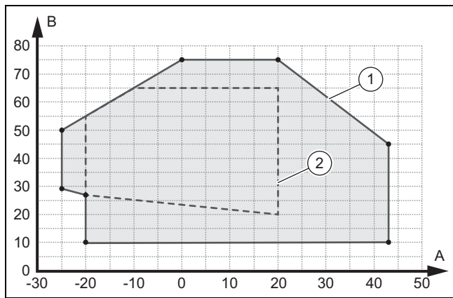
A Külső hőmérséklet B Fűtővíz-hőmérséklet 1 Fűtési üzem használhatósági határai 2 Alkalmazási terület a következő szerint: EN 14511
