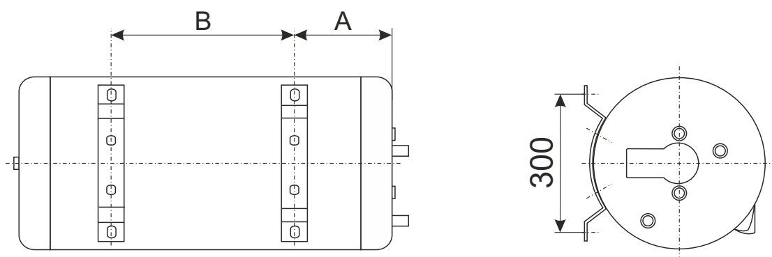
Slika 3. - Montaža kombiniranog bojlera LKB-Digi na zid
