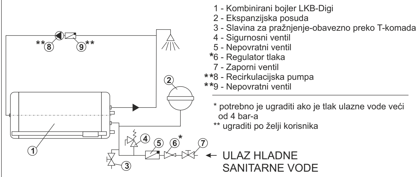
Shema 1. - Ugradnja kombiniranog bojlera LKB-Digi na vodovodnu instalaciju
