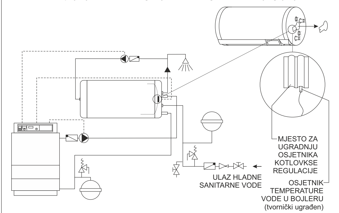
Shema 3. - Spajanje kombiniranog bojlera LKB-Digi na instalaciju grijanja
