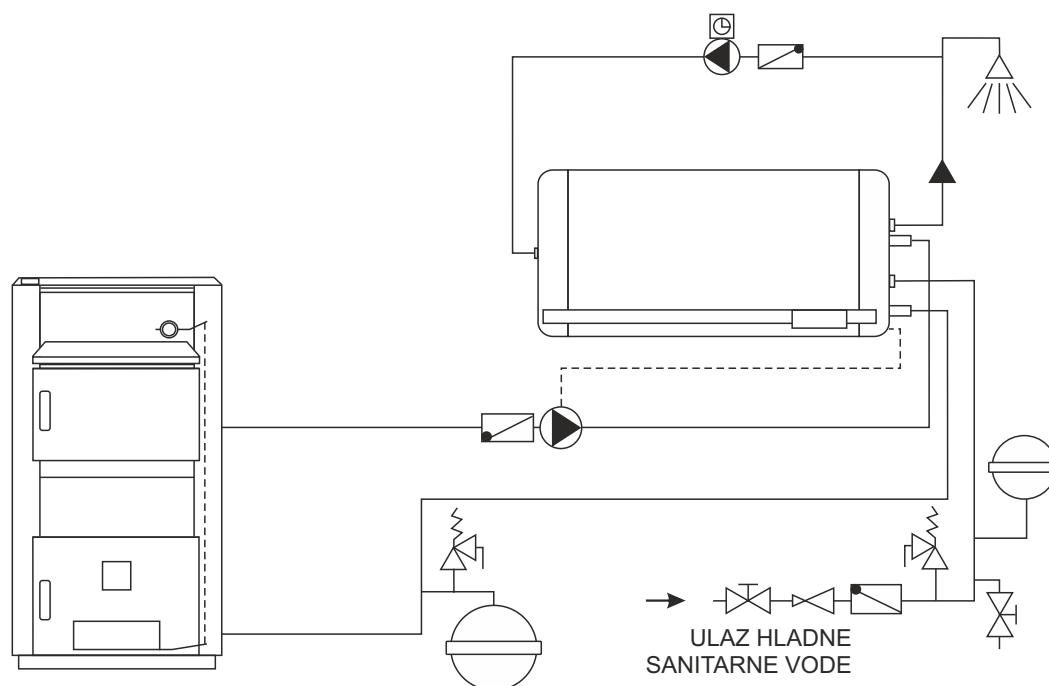
Shema 2. - Spajanje kombiniranog bojlera LKB-Digi na instalaciju grijanja
