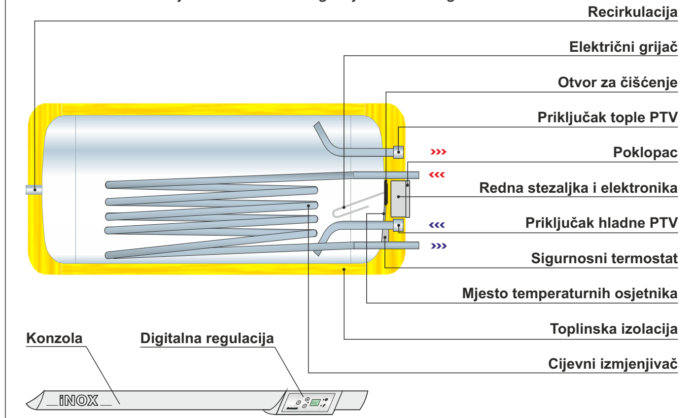
Slika 1. - Osnovni dijelovi kombiniranog bojlera LKB-Digi
