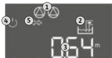
Fig. 29: Úvodní obrazovka: Snímač hladiny/ponorný zvon
