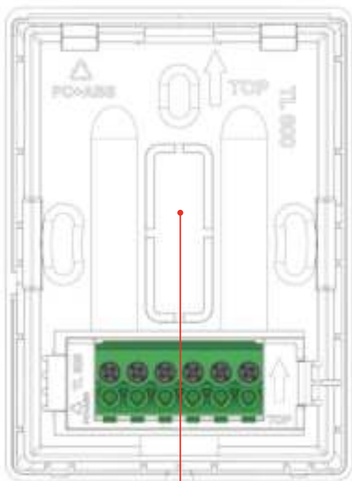
Odnímatelná část
