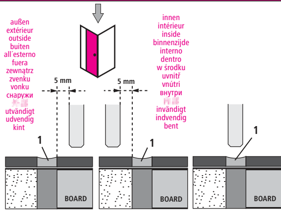
2 Versiegelung / Scellement / Sealing / Siliconen-kitnaad / Sigillatura / Sellado / Uszczelnienie zewnętrzne / Uzavirací náter / Tesniaca hmota / Герметик / Försigling / Försigling / Elzárás
