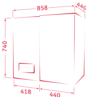
Sestava kotle Gepard Condens 12 / 25 MKO se zásobníkem VEQ 75/2 B umístěným vpravo
